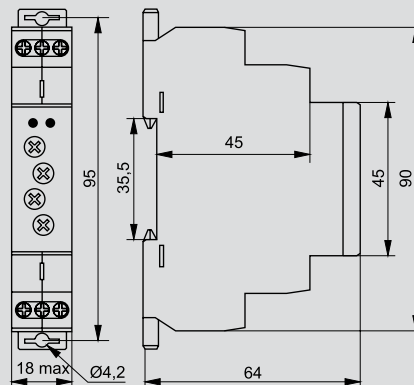
ORT. 2 конт.
