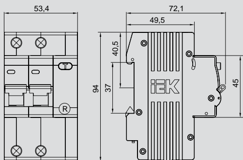
АД12S
