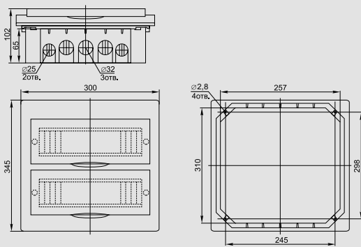
ЩРВ-П-24
