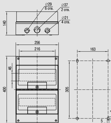
КМПн-24
