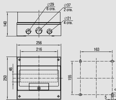
КМПн-12
