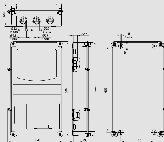
ЩУРН-П 3/12
