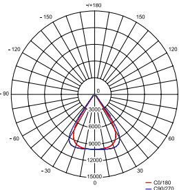
Тип Г (60°)
