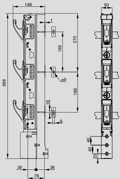
ПВР-1 160 А
