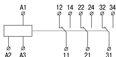
OIR-308 / OIR-316
